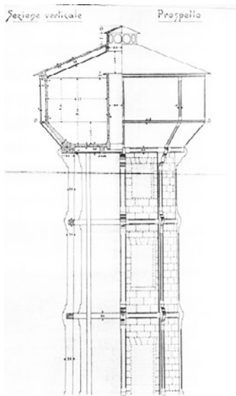
Disegno della cisterna a torre, mai realizzata
