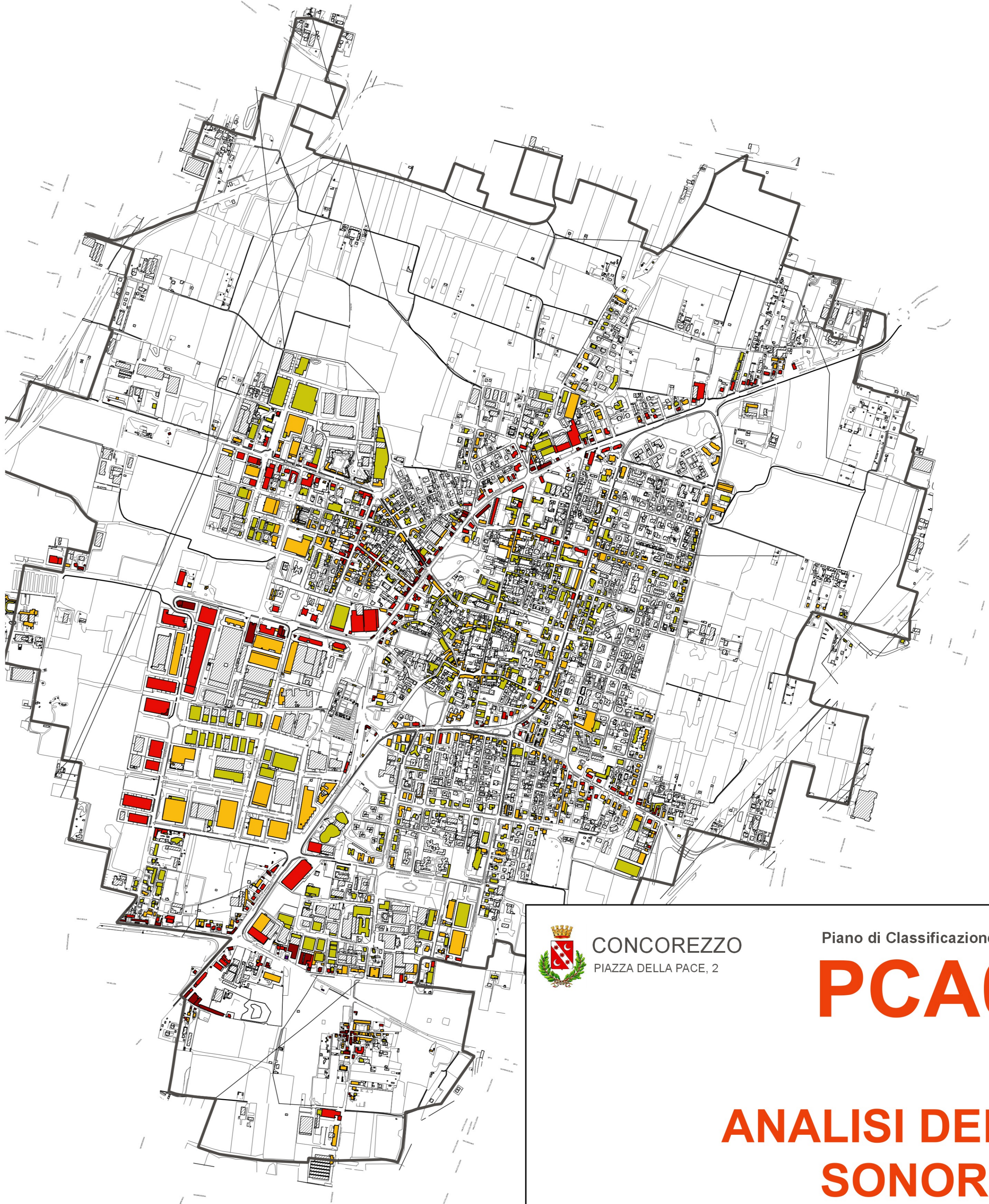
MAPPATURA ACUSTICA - LIVELLO NOTTURNO CORRISPONDENTE ALLA FACCIATA PIU' ESPOSTA
